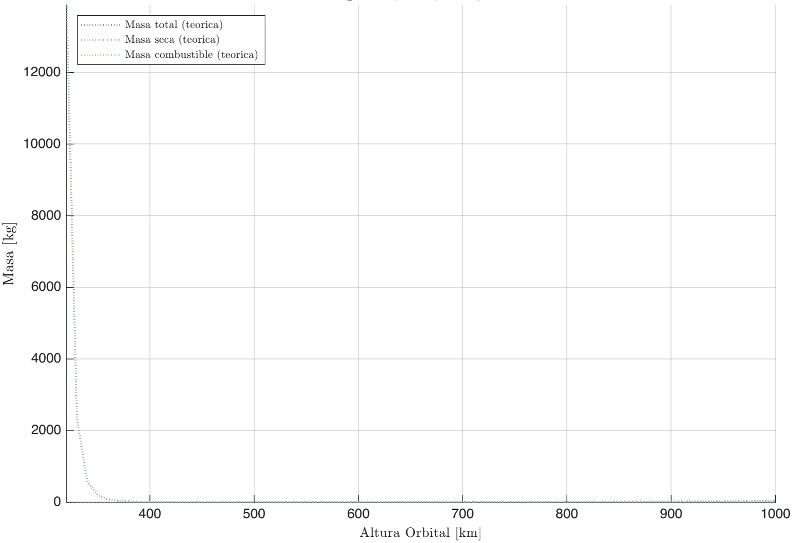
Desglose de Masas vs. Altura Config: 1 Sat, 1 Tel, Det 3, Korsch
